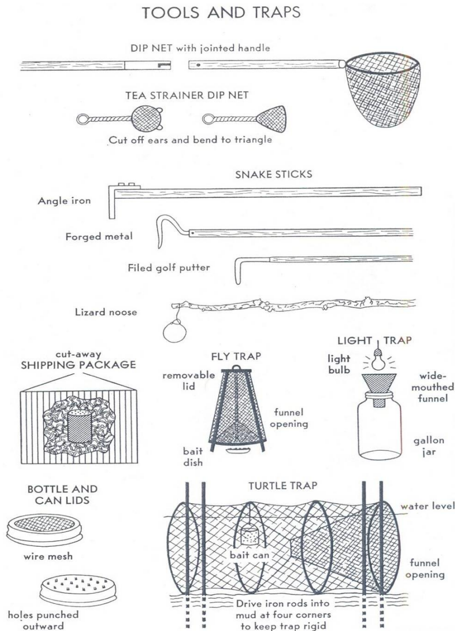
Figura 4. Algunos instrumentos y trampas para capturar anfibios y reptiles: redes, ganchos herpetológicos, lazos y nasas (tomado de Conant 1958).
