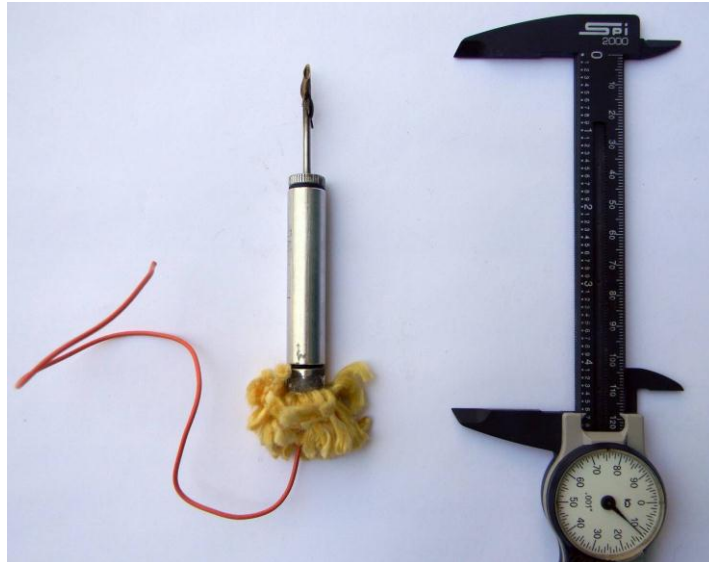
Figura 20.- Dardo tranquilizante equipado con radio transmisor. El radio transmisor permite que el animal al que fue disparado el dardo pueda ser rápidamente localizado (Fotografía L. Pérez-Solano).
