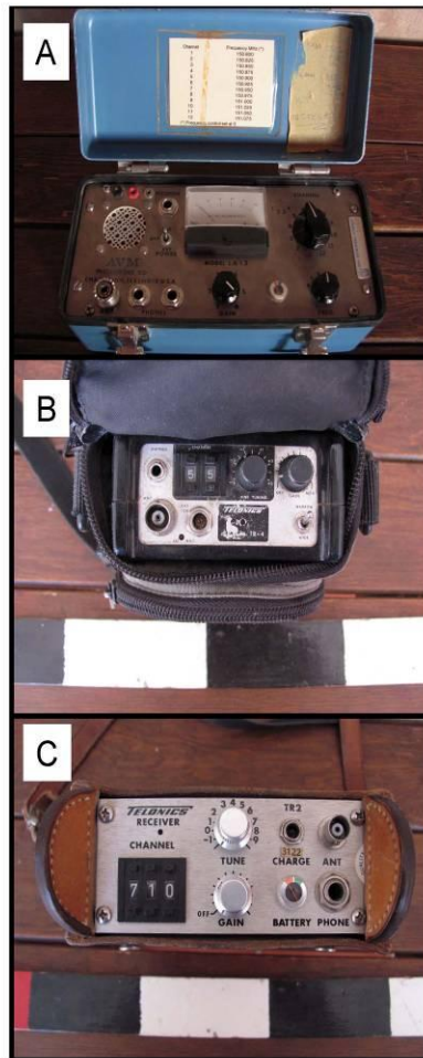
Figura 13.- Receptores de radio telemetría analógicos con capacidad de recibir: (A) 12 frecuencias de radio collares, (B) 99 frecuencias y (C) cientos de frecuencias. Las frecuencias a las cuales los receptores de la figuras A y B pueden recibir señales son programadas directamente por el fabricante a petición de los clientes (Fotografía M. Hidalgo).
