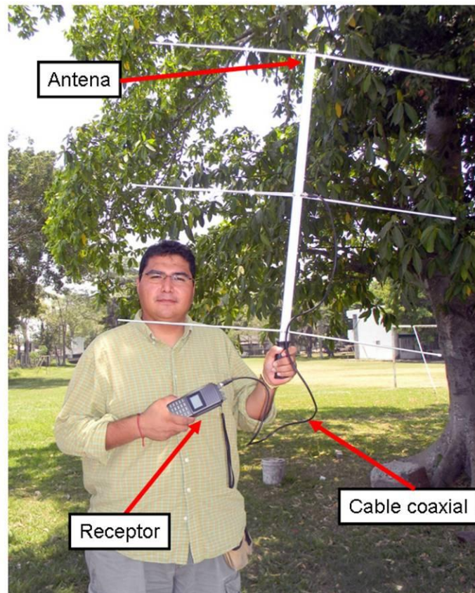
Figura 7.- Fotografía en la que se detallan los diferentes componentes del subsistema de recepción (Fotografía M. Hidalgo).
