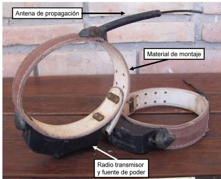
Figura 3.- Fotografía de un radio collar para carnívoro mediano en el cuál se detallan los diferentes componentes del subsistema de transmisión (Fotografía M. Hidalgo).
