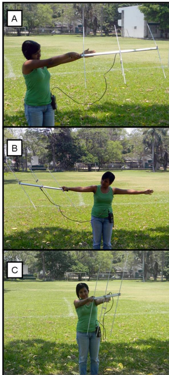
Figura 16.- Procedimiento estándar para obtener la dirección de un radio transmisor utilizando una antena Yagui. A. – Una vez que se escucha la señal del radio transmisor, se busca cual es el punto donde se tiene la mayor ganancia. Una vez hecho esto, se reduce la ganancia y el volumen del receptor al mínimo, y se comienza a mover la antena hasta que se deje de escuchar la señal emitida por el radio transmisor. Con un brazo se marca la dirección donde se deja de escuchar la señal. B. – Se mueve la antena hacia el lado contrario con el objetivo de buscar la dirección donde se deja de escuchar la señal emitida por el radio transmisor en ese lado del área de recepción de la antena. Se marca esta nueva dirección con el otro brazo. C. – Se cierran ambos brazos a la misma velocidad con el objetivo de marcar con la antena la dirección mas probable en la que se encuentra el radio transmisor.
