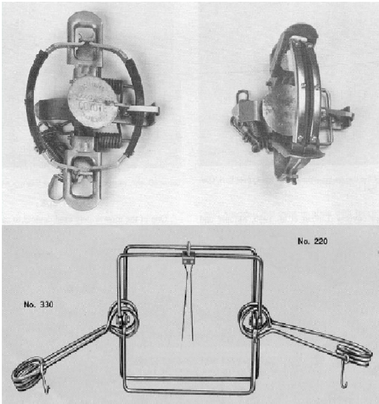
Figura 1. Arriba cepos suave "Victor" (esta trampa presenta un recubrimiento de neopreno para evitar el daño a los animales. Abajo trampa "Conibear" para sujetar del cuerpo, ésta es letal.
