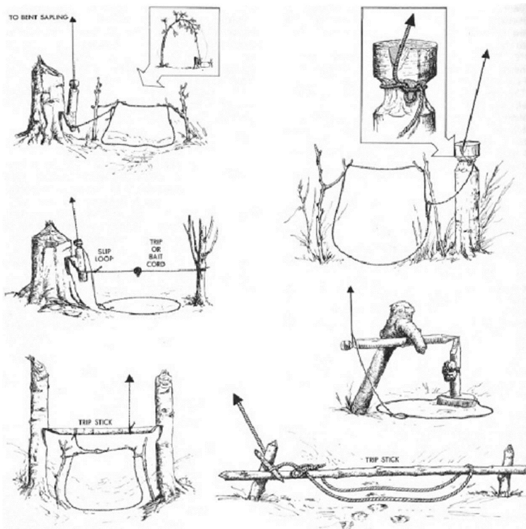
Figura 5. Diferentes formas de colocar los lazos matreros.
