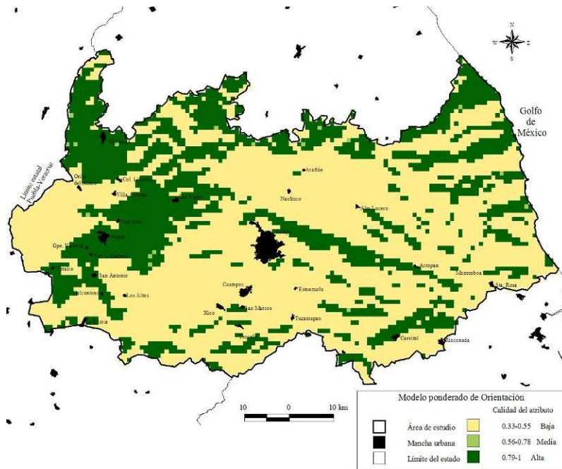
Modelo de orientación de las laderas generado a partir del MDE del Hydro1k del USGS
