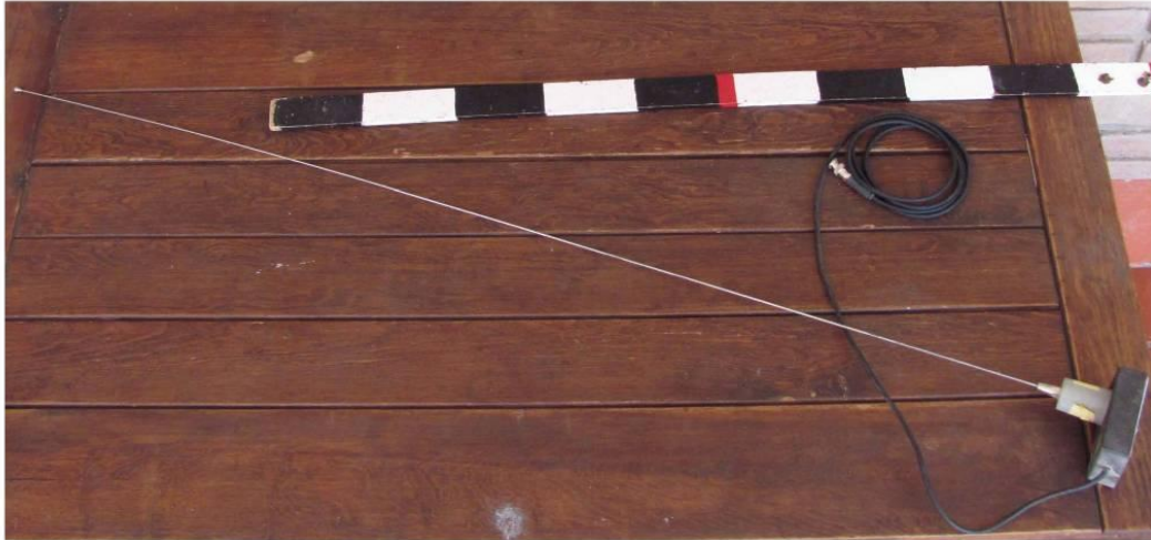
Figura 8.- Antena de recepción de dipolo o de látigo colocada en posición horizontal. La base de la antena tiene un poderoso imán que permite ser colocada en el techo de un vehículo. Cada una de las divisiones blancas y negras de la regla de referencia corresponden a 10cm (Fotografía M. Hidalgo).
