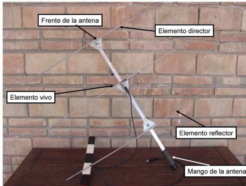
Figura 10.- Antena Yagui de tres elementos en la que se destacan sus diferentes partes. El elemento vivo es el sitio donde se concentra la señal para ser enviada al receptor a través del cable coaxial. En las antenas con un mayor número de elementos, todos los elementos adelante del elemento vivo se llaman directores, mientras que todos los que se encuentran atrás se llaman reflectores. Es importante que las antenas cuenten con un mango aislante para que la persona que sostiene la antena no produzca interferencia en la recepción de la señal y como consecuencia disminuya la ganancia de la antena (Fotografía M. Hidalgo).
