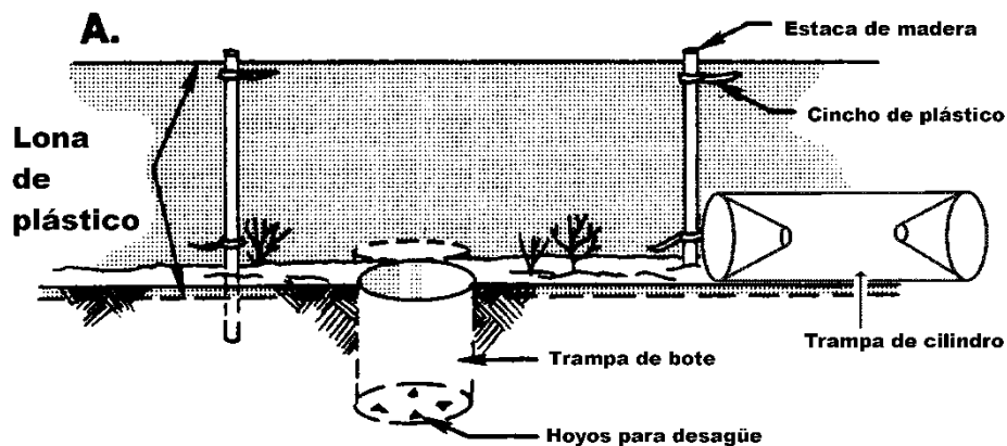
Figura 7. Trampa terrestre de cerco de desvío en combinación con trampas de fosos (bote) y de cilindro (modificado de Heyer et al. 2001).
