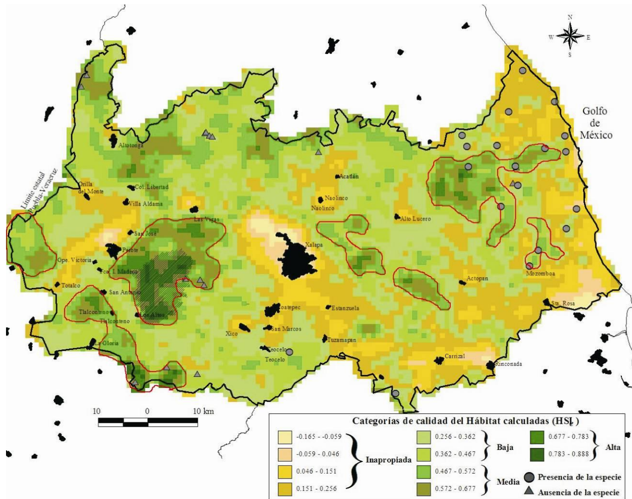
Figura 8. Modelo del HSI calculado, donde se muestran las áreas seleccionadas según su amplitud y calidad como potenciales áreas de manejo para la especie (líneas rojas) y los sitios de muestreo (tomado de Delfín-Alfonso et al. 2009).
