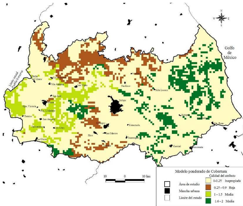
Modelo de cobertura generado a partir del imágenes de satélite Landsat con el apoyo del mapa de uso del suelo y vegetación.
